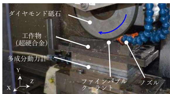
平面研削盤の写真
